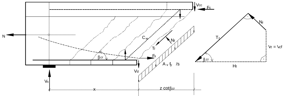
Figura 1.1 – Mecanismos de transferencia de cortante (adaptada de Reineck, 1991a)
