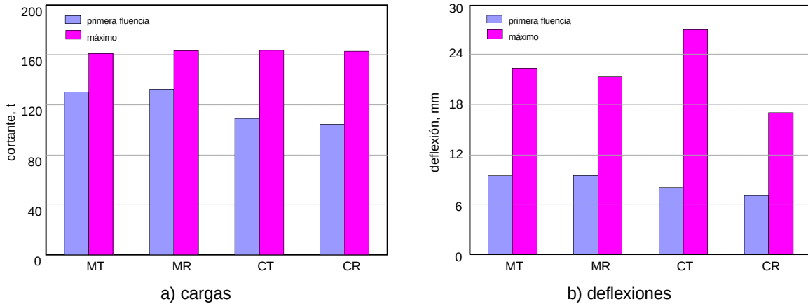
Figura 8.5 – Cargas y deflexiones asociadas a la primera fluencia y a la resistencia
