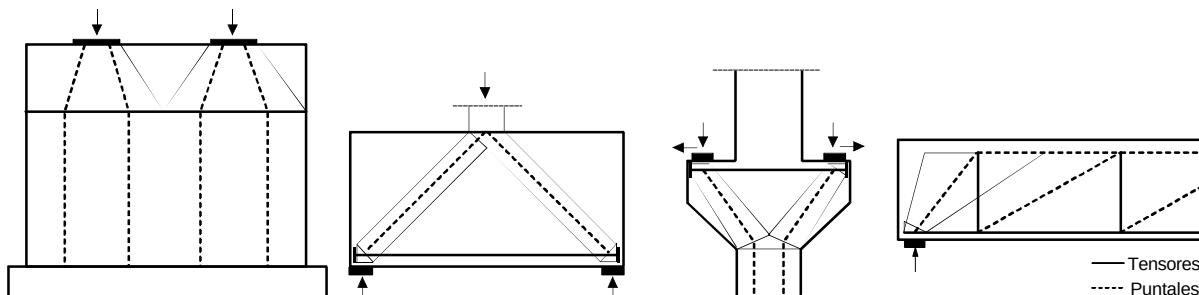
Figura 2.1 – Elementos modelados con puntales y tensores
