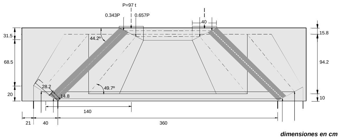
Figura 3.2 – Modelo de puntales y tensores empleado
