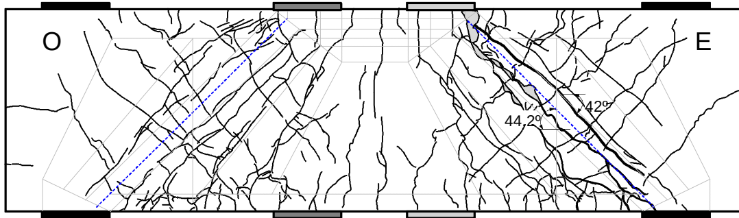
Figura 6.9 – Orientación del puntal de compresión (modelo CT)
