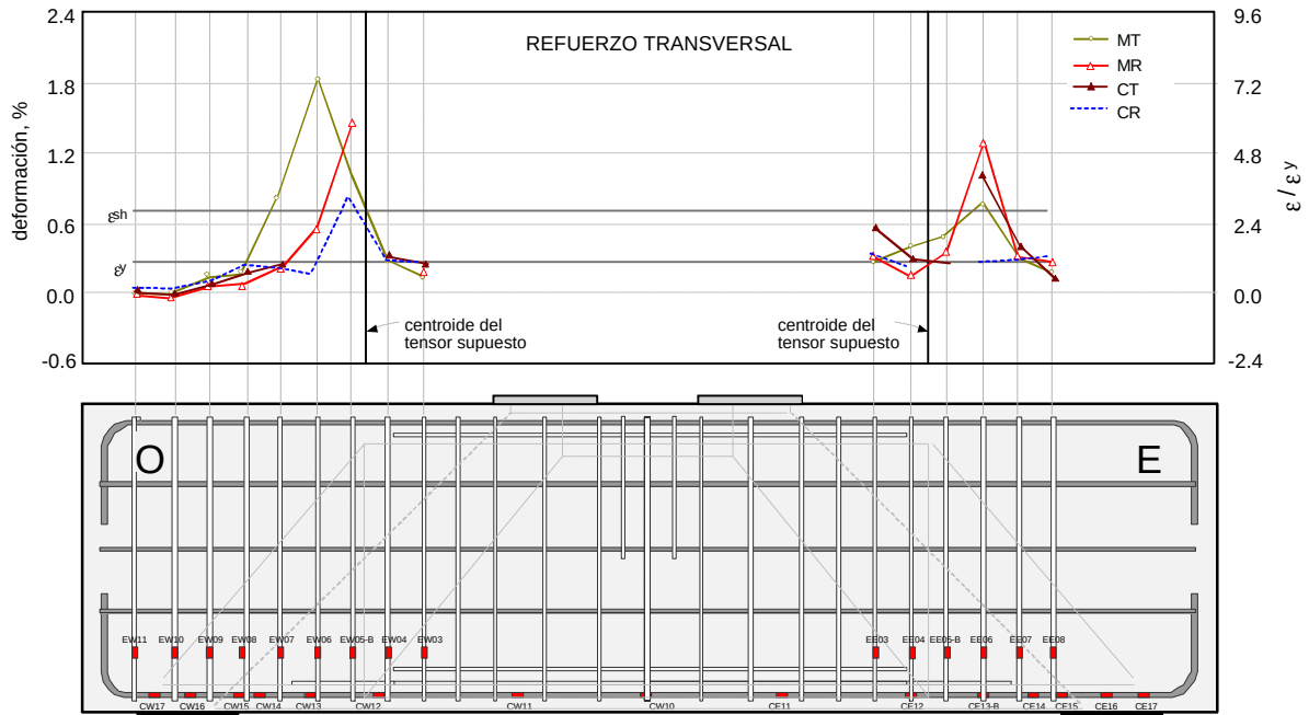
Figura 8.22 – Deformaciones en el refuerzo transversal de los especímenes ensayados al alcanzar su resistencia
