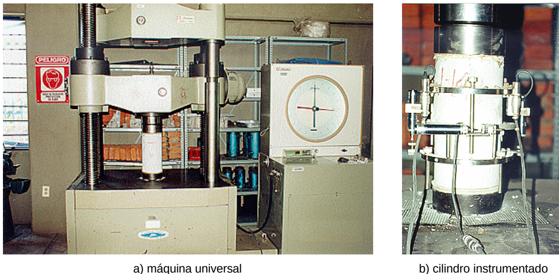
Figura A.2 - Ensaye de compresión de un cilindro de concreto
