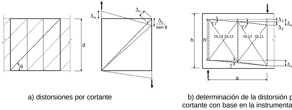
Figura 4.2 – Distorsiones por cortante en el alma de una viga de concreto reforzado
