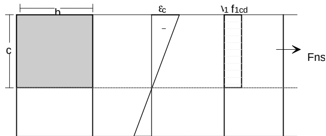
Figura 2.13 – Resistencia de un puntal de compresión prismático ( Fédération , 1998)
