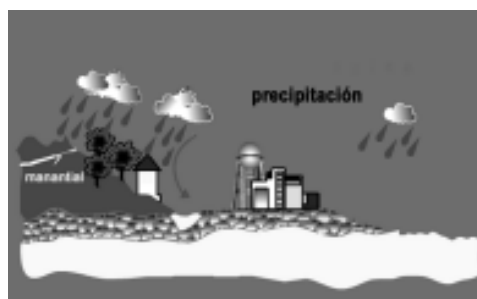
c) Precipitación
