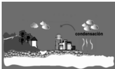
b) Condensación
