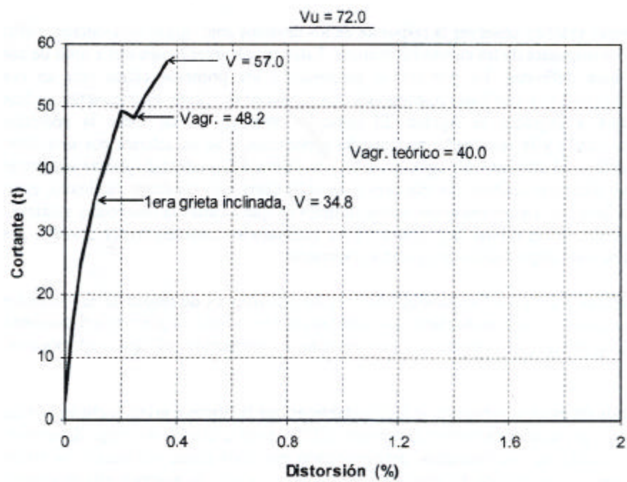
Figura 3.37 Modelo M-250R: Envolvente de respuesta ( 1\ t = 9.81\ kN )
