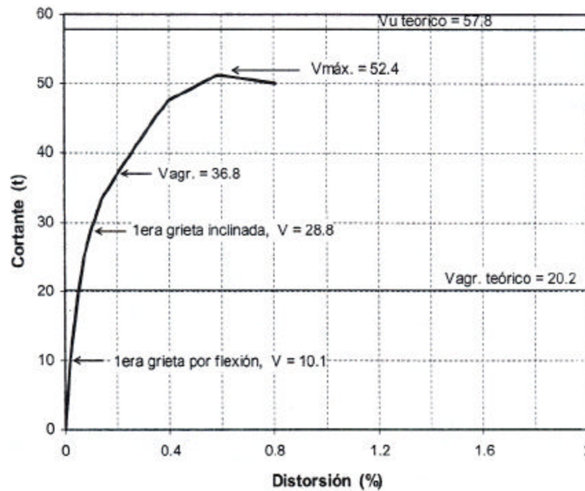
Figura 3.40 Modelo M-211: Envolvente de respuesta ( 1 \text{ t} = 9.81 \text{ kN} )
