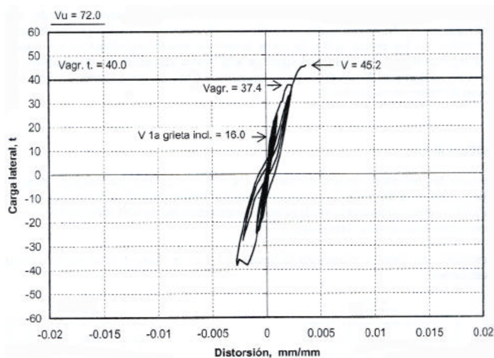
Figura 3.16 Curva histerética del modelo M-250 ( 1\text{ t} = 9.81\text{ kN} )
