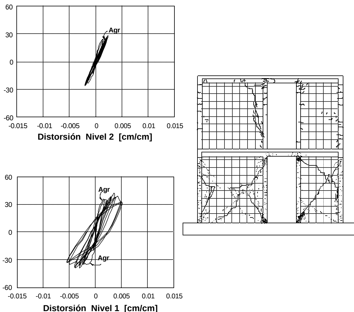
Figura 1.12 Curvas histeréticas y patrón de agrietamiento final del modelo 3D
