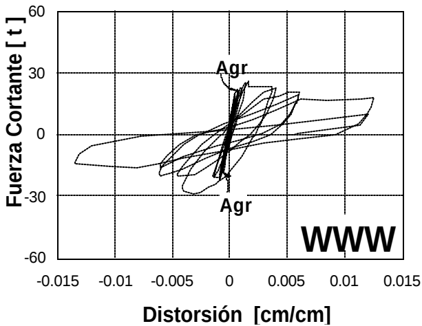
Figura 1.8 Resultados de la fase uno: Curvas de histéresis y patrones de agrietamiento final
