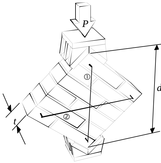
Figura 1.17 Pruebas de corte en muretes de mampostería
