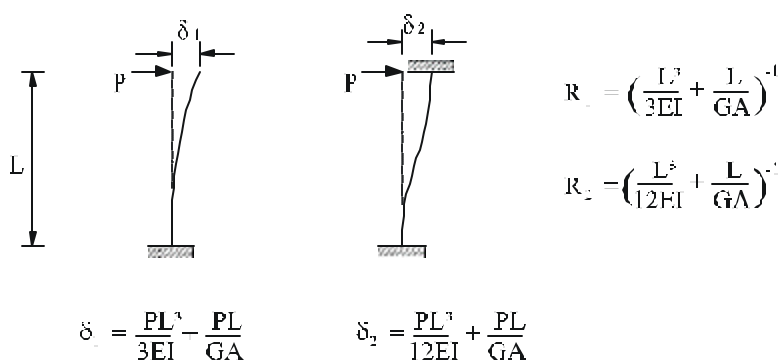
Figura A.4 Rangos en que varía la rigidez de una columna ancha ante desplazamiento lateral según su condición de borde
