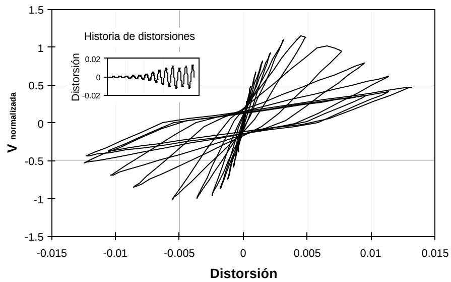
Figura 2.11 Respuesta histerética calculada para una historia de distorsiones senoidal creciente
