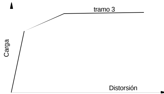
Figura 4.2 Envolvente cortante-desplazamiento para muros usada en LARZ
