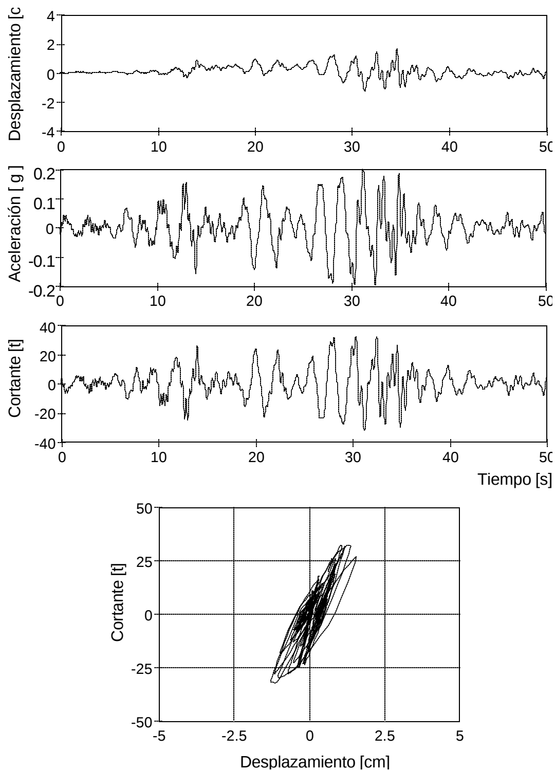
Figura 3.9 Resultados del análisis paso a paso usando el modelo histerético para muros de mampostería confinada sin refuerzo horizontal
