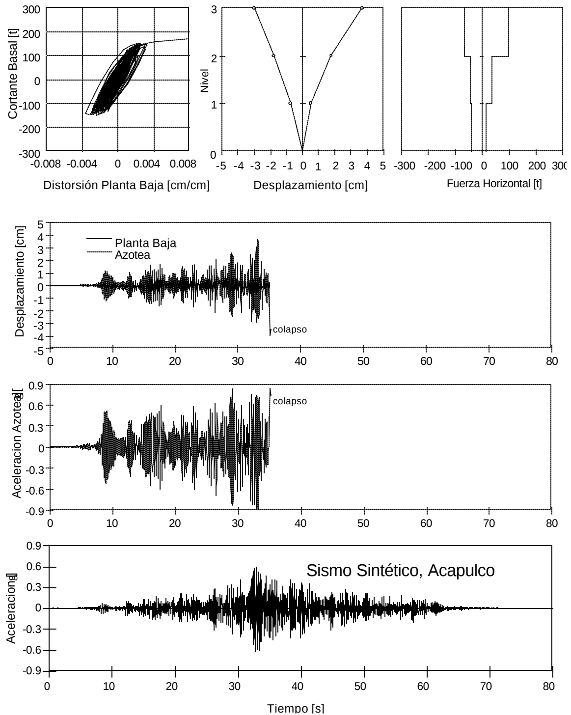
Figura 5.7 Resultados del análisis de la estructura 3A 1 SR
