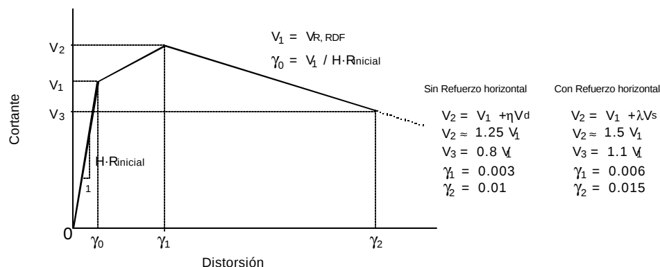
Figura 3.2 Envolvente propuesta para el modelo histérico
