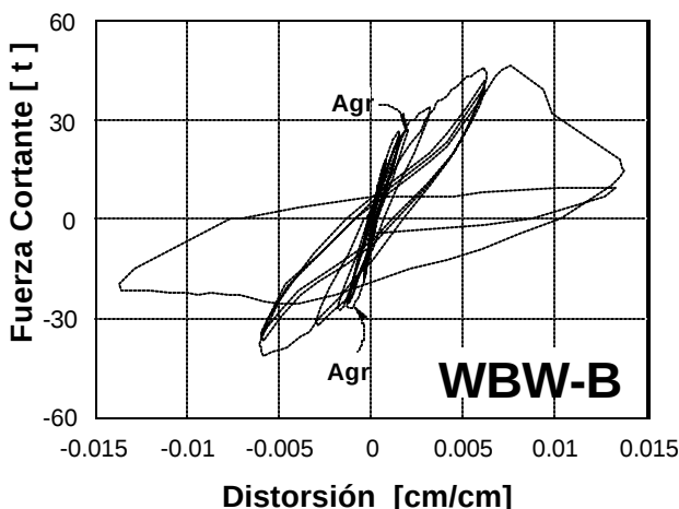
Figura 1.10 Curvas de histéresis y patrones de agrietamiento final de la segunda fase
