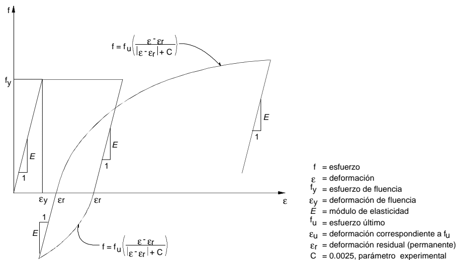
Figura 4.1 - Curva esfuerzo-deformación idealizada para el comportamiento del acero de refuerzo grado 42 ante carga cíclica
