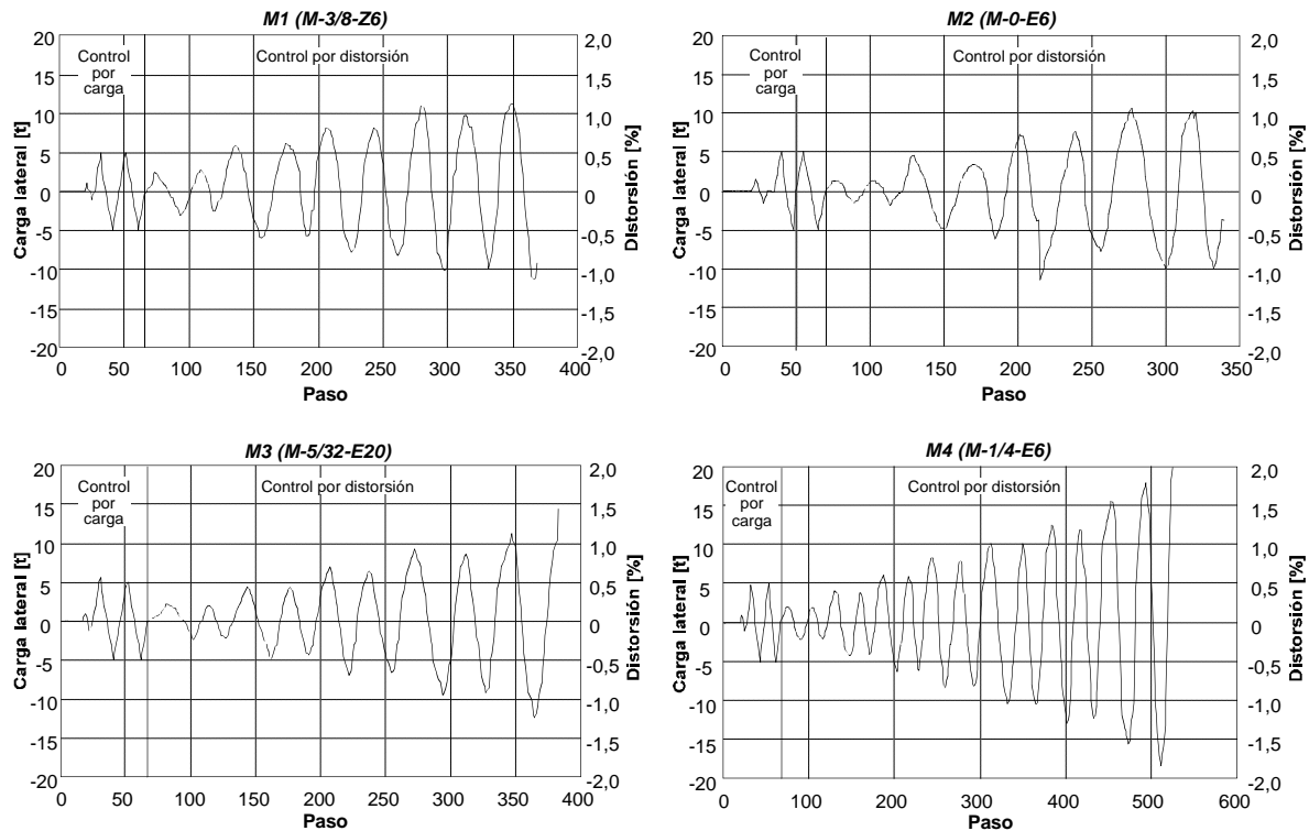
Figura 2.6 - Historias de carga
