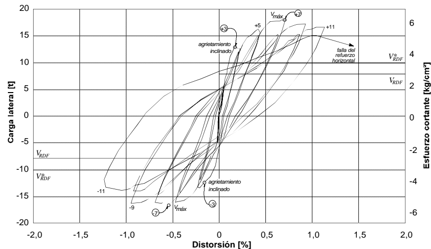
Figura 3.30 - Curva carga lateral-distorsión del espécimen M3 (M-5/32-E20)
