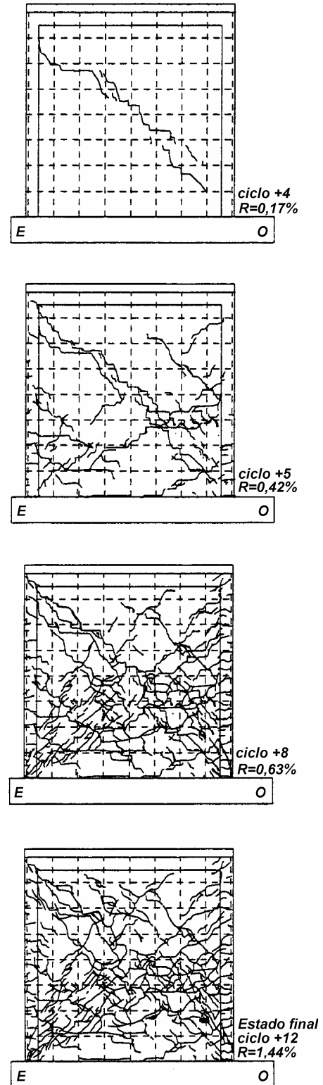
Figura 3.28 - Evolución del agrietamiento durante el ensaye del espécimen M3 (M-5/32-E20)
