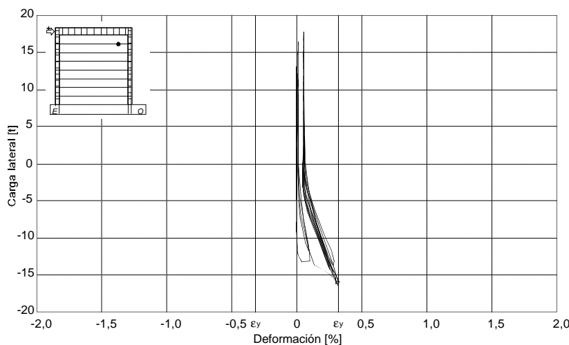
Figura 4.21 - Deformación en el extremo Oeste de uno de los alambres del refuerzo horizontal del espécimen M3 (deformímetro B07)
