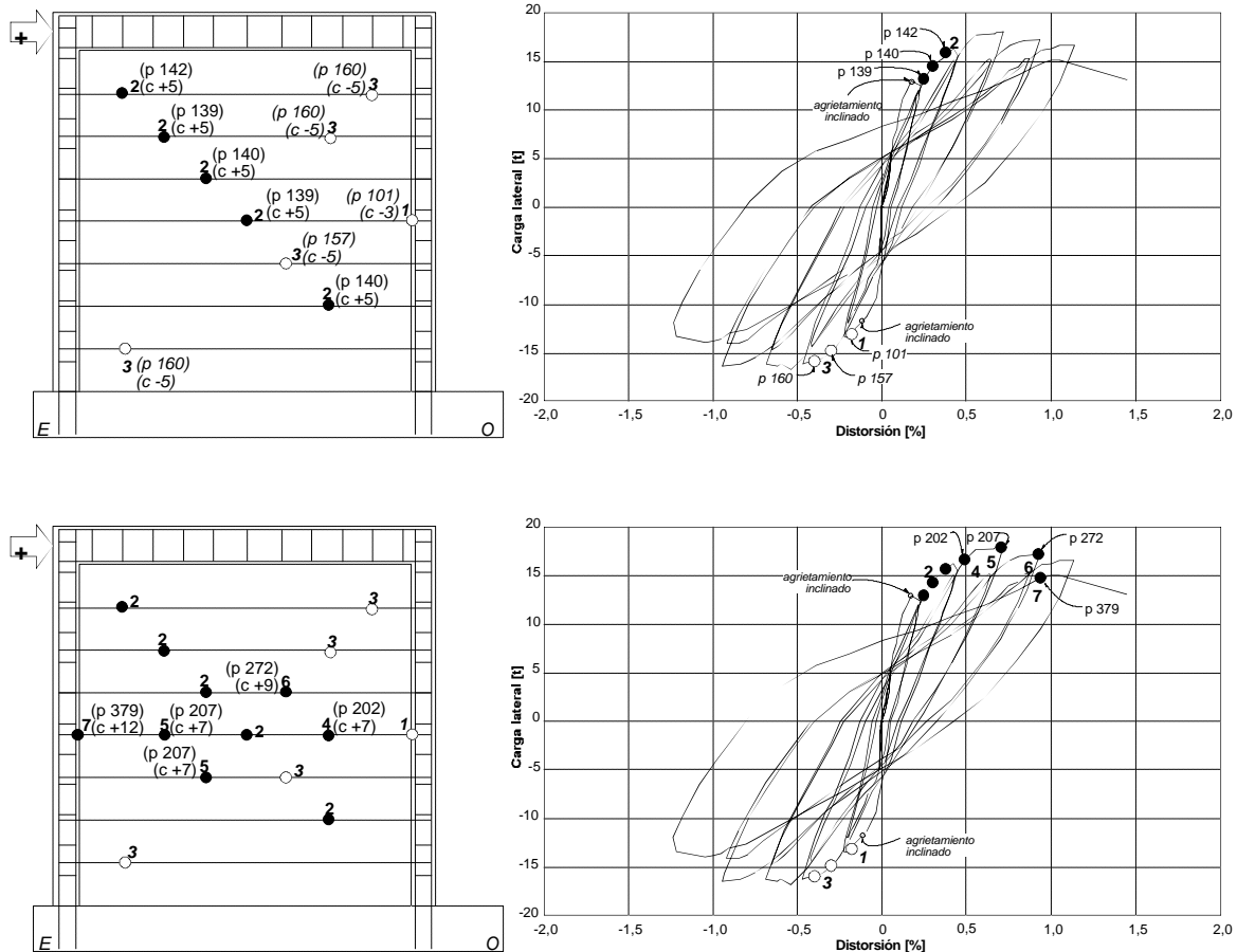
Figura 4.19 - Secuencia de fluencia del refuerzo horizontal del espécimen M3 (M-5/32-E20)
