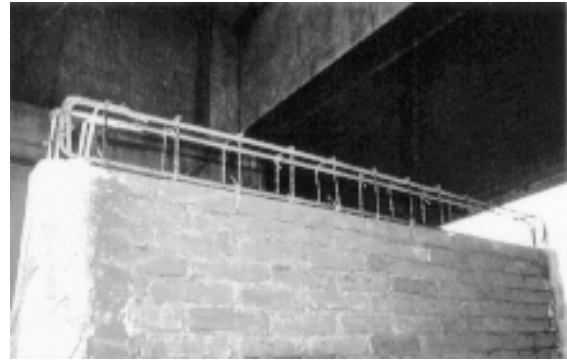
d) Armado de dala de M2
