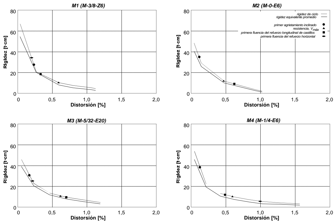
Figura 5.7 - Degradación de rigidez de ciclo y de rigidez equivalente de los especímenes ensayados
