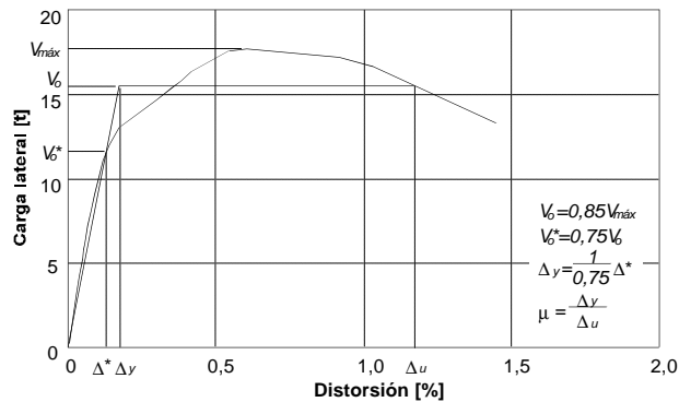
Figura 5.12 - Cálculo de la ductilidad de acuerdo con el criterio de Park
