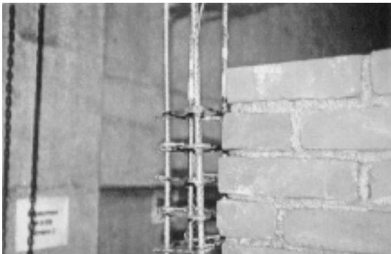
c) Armado de castillos de M2
