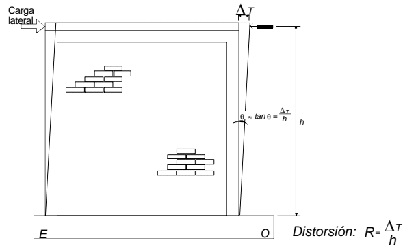
Figura 3.1 - Definición de distorsión
