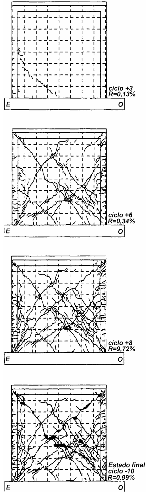
Figura 3.19 - Evolución del agrietamiento durante el ensaye del espécimen M2 (M-0-E6)
