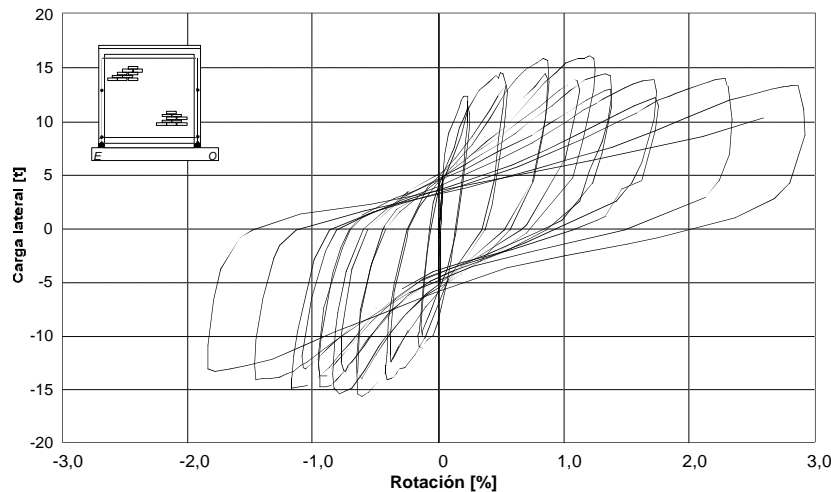
Figura 3.40 - Rotación local promedio en la base de los castillos del espécimen M4 (M-1/4-E6)
