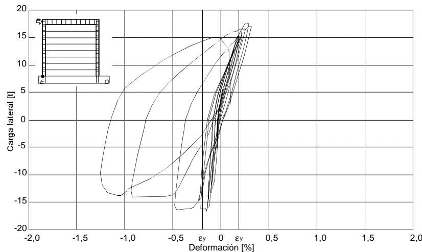
Figura 4.17 - Deformación en la base del castillo Este del espécimen M3 (deformímetro CEL1)
