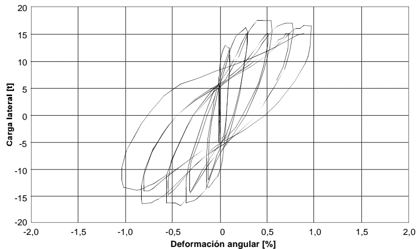
Figura 3.33 - Deformación angular del panel de mampostería del espécimen M3 (M-5/32-E20)
