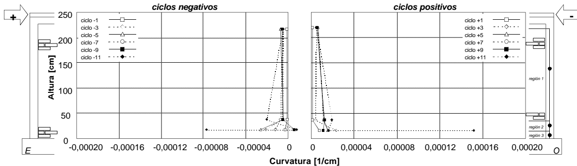
Figura 3.13 - Distribución de curvaturas en la altura del espécimen M1 (M-3/8-Z6)
