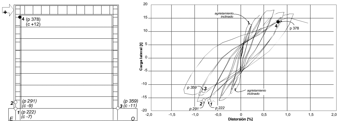
Figura 4.16 - Secuencia de fluencia del refuerzo de castillos del espécimen M3 (M-5/32-E20)
