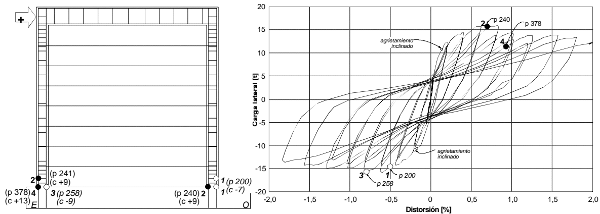
Figura 4.25 - Secuencia de fluencia del refuerzo de castillos del espécimen M4 (M-1/4-E6)
