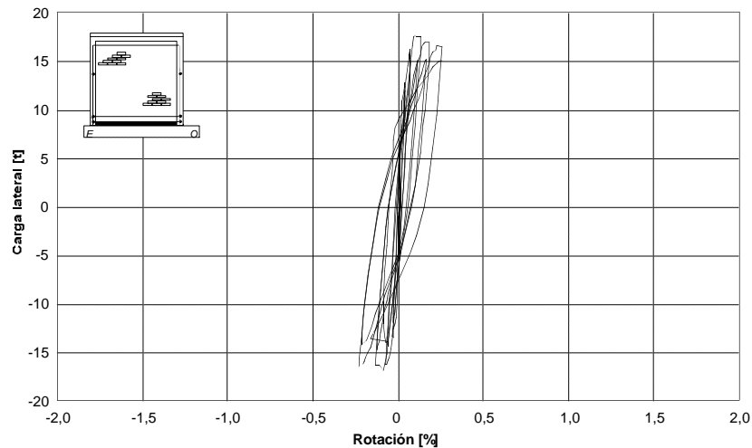
Figura 3.31 - Rotación del espécimen M3 (M-5/32-E20) en la región 3
