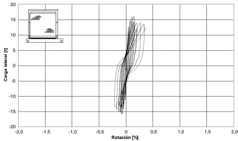
Figura 3.39 - Rotación del espécimen M4 (M-1/4-E6) en la región 3
