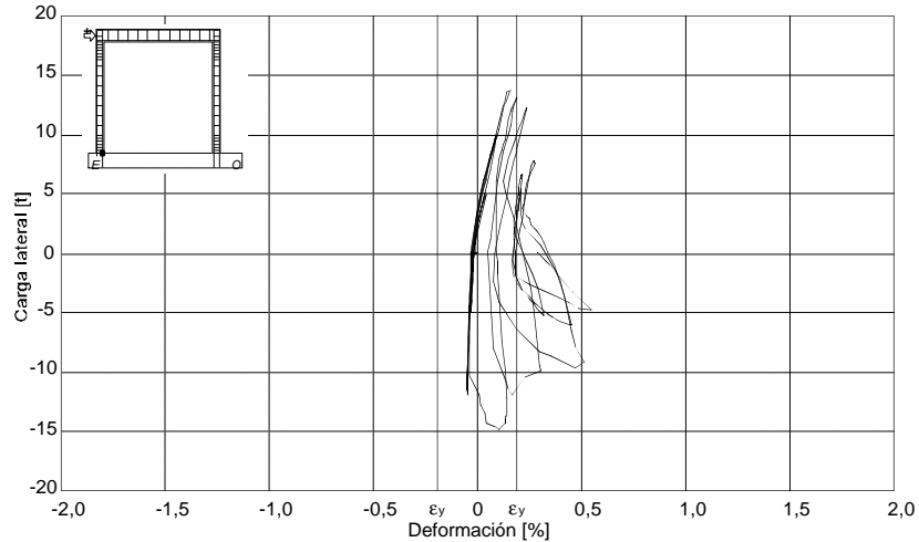
Figura 4.13 - Deformación en la base del castillo Este del espécimen M2 (deformímetro CEL2)
