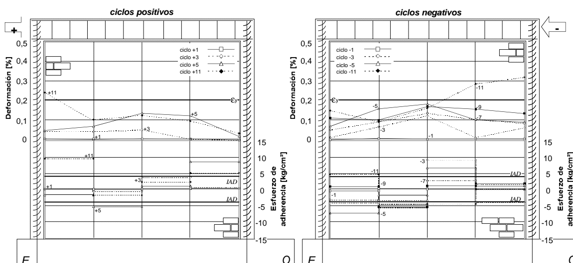
Figura 4.9 - Deformación y esfuerzo promedio de adherencia a lo largo de la barra central del espécimen M1 (M-3/8-Z6)
