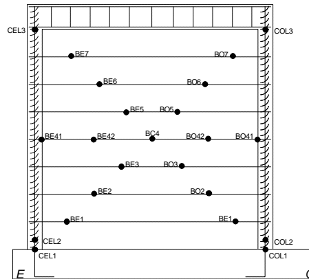
Figura 4.3 - Instrumentación interna del espécimen M1 (M-3/8-Z6)
