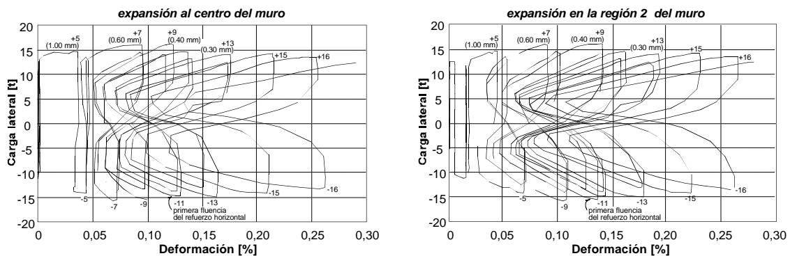
Figura 3.42 - Expansiones del espécimen M4 (M-1/4-E6)
