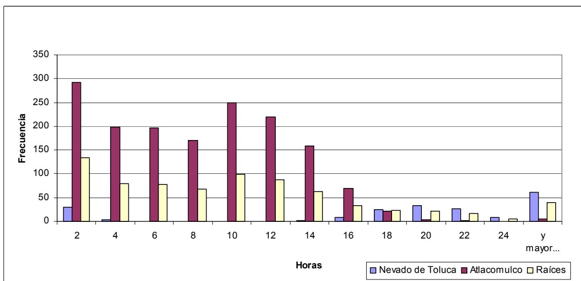
Figura 12 Frecuencias de ondas menores o iguales a 10°C del Nevado de Toluca, Atlacomulco y Raíces
