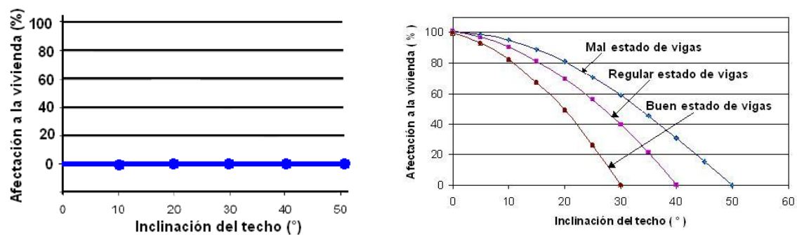
Figura 25 Función de vulnerabilidad para casas con techos de losa de concreto (izquierda) y para viviendas con techos de lámina en lugares donde puede ocurrir una nevada (derecha)
