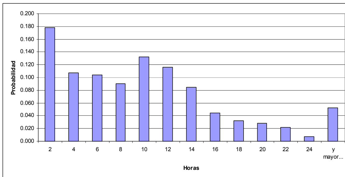
Figura 14 Probabilidad de duración de onda de baja temperatura menor o igual a 10°C y mayores a 5°C en Raíces
