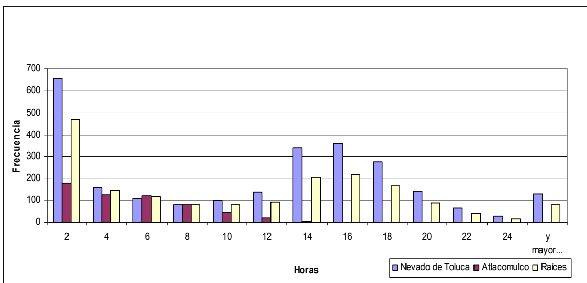
Figura 13 Frecuencias de ondas menores o iguales a 5° C y mayores a 0° C del Nevado de Toluca, Atlacomulco y Raíces
